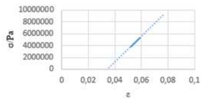
Linearni dio krivulje naprezanje – deformacija za uzorak 2P4
