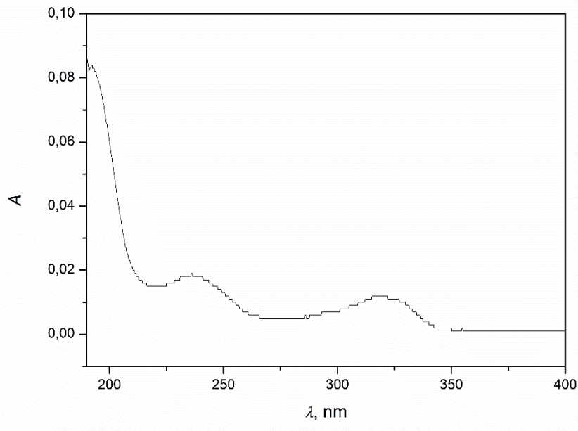
Slika 16. Apсорpcijski spektar pomoćnih tvari u acetonitrilu
