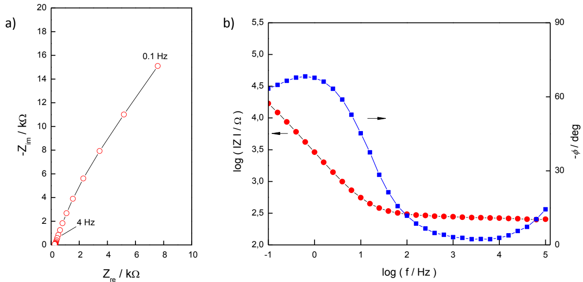
Slika 4.2.3.4. Prikaz EIS rezultata dobivenih za Pt elektrodu na koju je nanesen rGO(OMW, pH=10) pri potencijalu -200 mV a) Nyquistov dijagram, b) Bodeov dijagram
