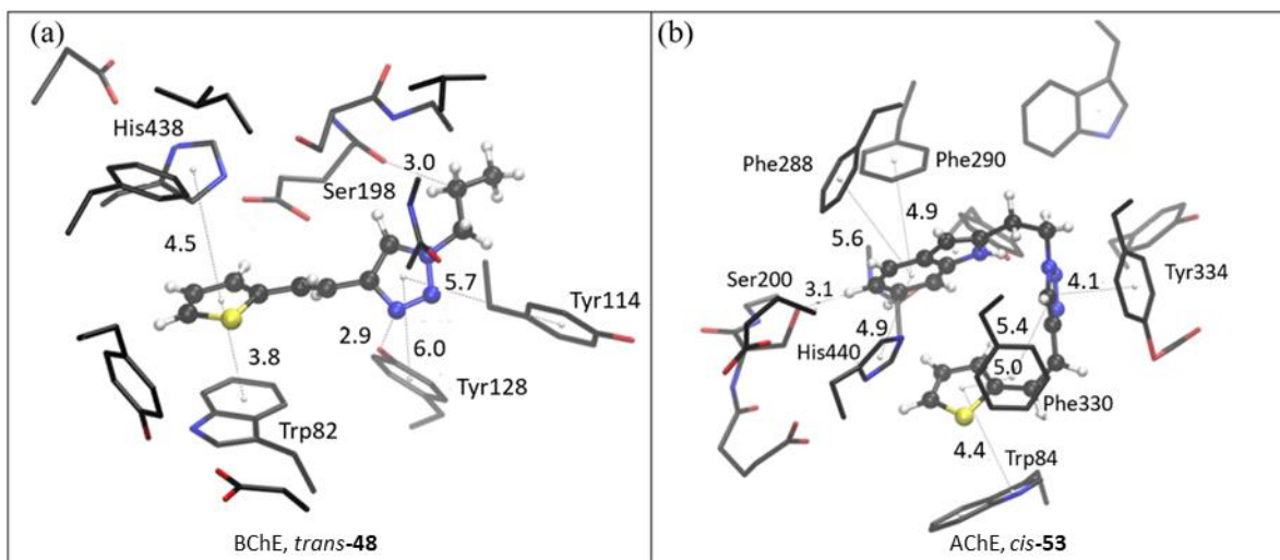
Slika 68. Strukture aktivnog mjesta BChE i trans - 48 (a) i AChE i cis - 53 (b). Molekule potencijalnih inhibitora prikazane su pomoću modela kuglica i štapića.
