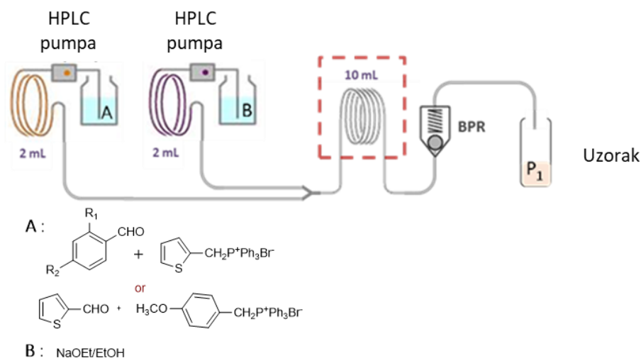
Slika 149. Milireaktorski sustav za Wittigovu reakciju dobivanja 128 , 215-217 [301].
