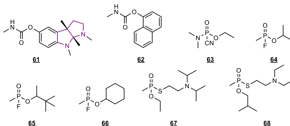
Slika 16. Strukture ireverzibilnih inhibitora kolinesteraza (karbamatni i organofosforini spojevi 61-68) [181].
