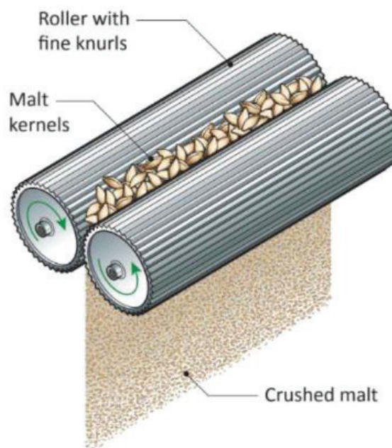
Slika 3; dvovaljak mlina
