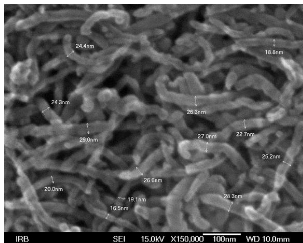
Slika 27. Prikaz uzorka 1 snimljenog SEM-om pri povećanju od 150000 puta.
