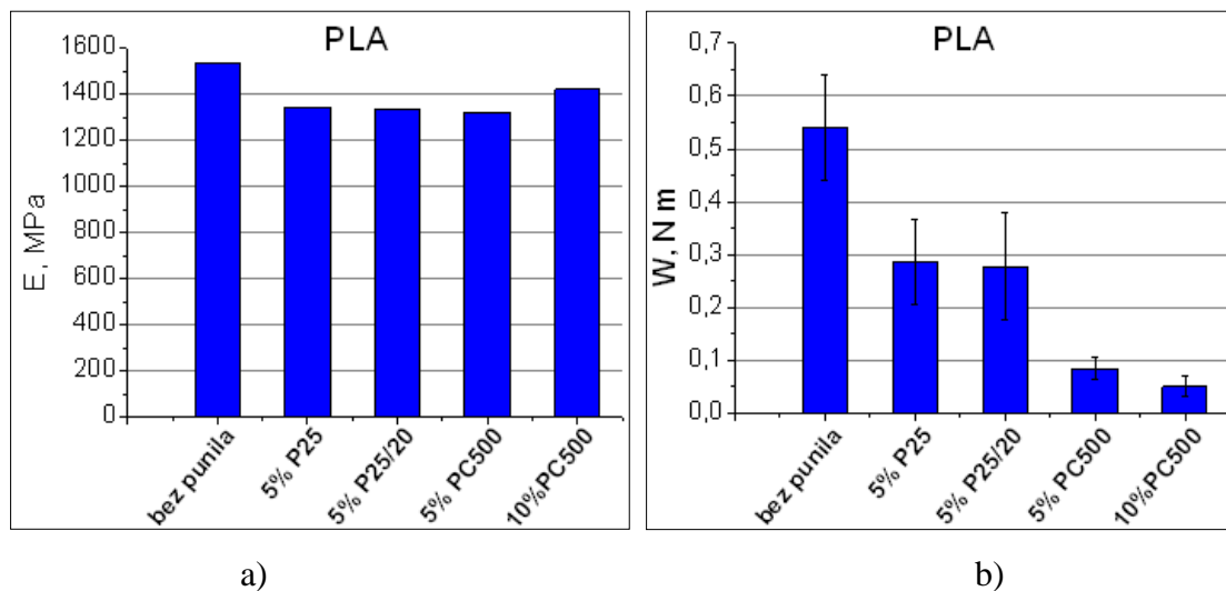
Slika 35: Usporedba mehaničkih svojstava čistog PLA i nanokompozita PLA: Youngov modul (a); rad loma (b)
