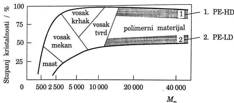
Slika 17: Utjecaj molekulne mase i stupnja kristalnosti na konzistenciju polietilena 5
