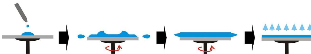
Slika 8. Prikaz oblaganja rotacijom [49]
