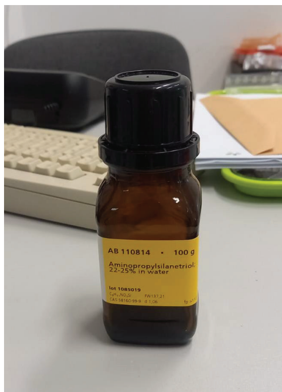
Slika 9. Aminopropilsilanetriol
