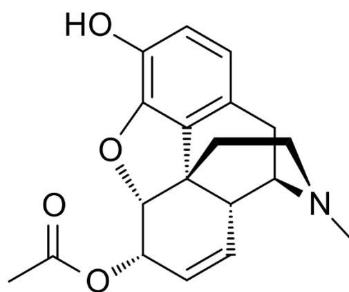
Slika 12. 6-monoacetilmorfin [33]
