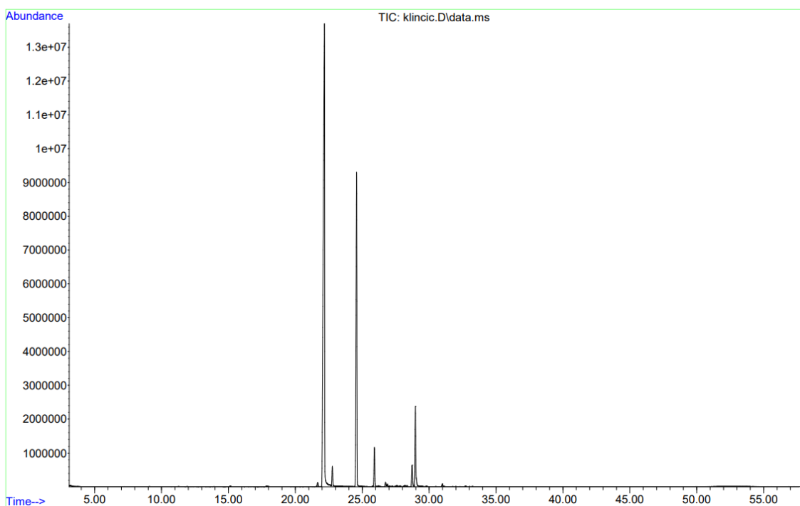
Slika 24. Kromatogram uzorka eteričnog ulja klinčića ( Syzgium aromaticum )
