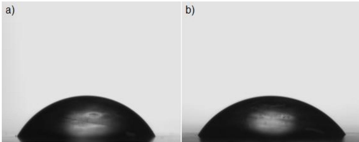
Slika 17. Kontaktni kut vode za komercijalnu (a) i modificiranu (b) DK membranu
