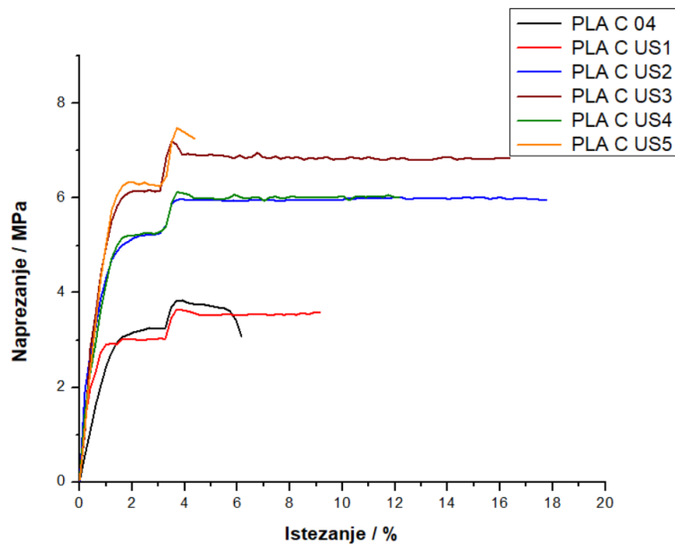
Slika 26. Dijagram napreznje-isteznje uzoraka sustava PLA C kojima je varirano vrijeme miješanja s ultrazvučnim homogenizatorom:
