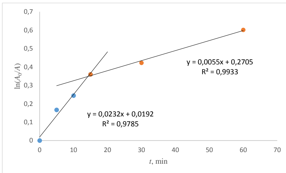
Slika 28. Kinetika fotolitičke razgradnje albendazola pri UV-C zračenju
