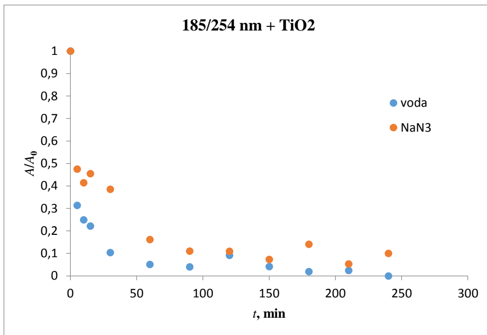
Slika 39. Fotokatalitička razgradnja albendazola sa i bez NaN 3 uz UV-C zračenje
