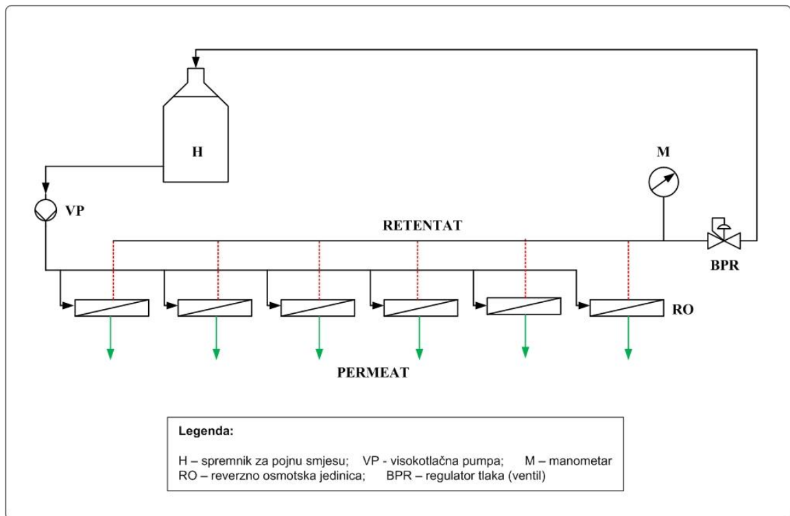
Slika 2. Shema laboratorijskog RO/NF uređaja
