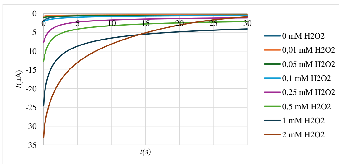
Slika 57: Kronoamperogrami u otopinama \text{H}_2\text{O}_2 različitih koncentracija snimljeni na -0,1 \text{ V} na sitotiskanoj elektrodi (20 min)
