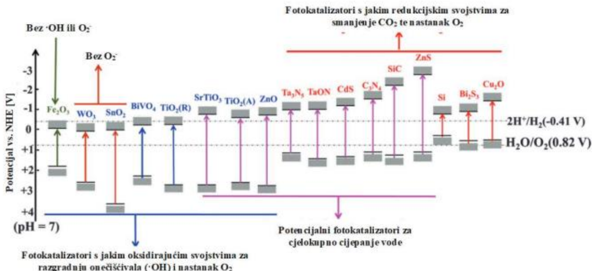
Slika 3.4. Moguća primjena određenih fotokatalizatora
