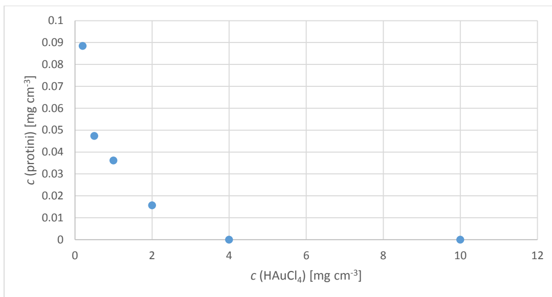
Slika 17. Utjecaj različitih koncentracija \text{HAuCl}_4 na sintezu nanočestica (redestilirana voda, c(\text{K}_2\text{CO}_3) = 1 \text{ mM} , T = 37 \text{ }^\circ\text{C} , 150 \text{ rpm} , c_{\text{ureaze}} = 2 \text{ mg cm}^{-3} , t = 24 \text{ h} , V = 10 \text{ cm}^3 )
