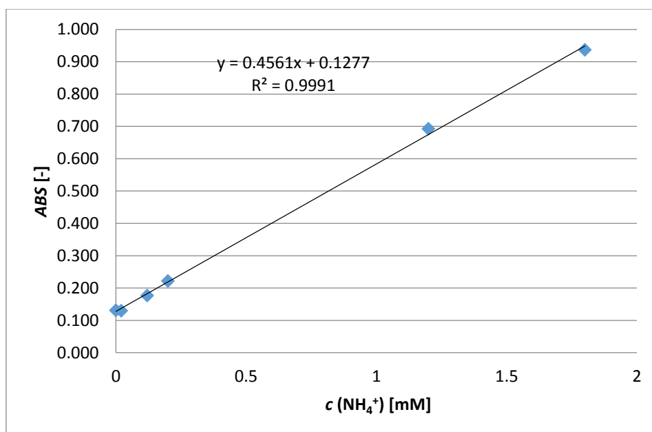
Slika 35 Baždarni dijagram za određivanje koncentracije amonijevih iona ( c(\text{NH}_4\text{Cl}) = 0 -2,0 \text{ mM} ; \lambda = 685 \text{ nm} )
