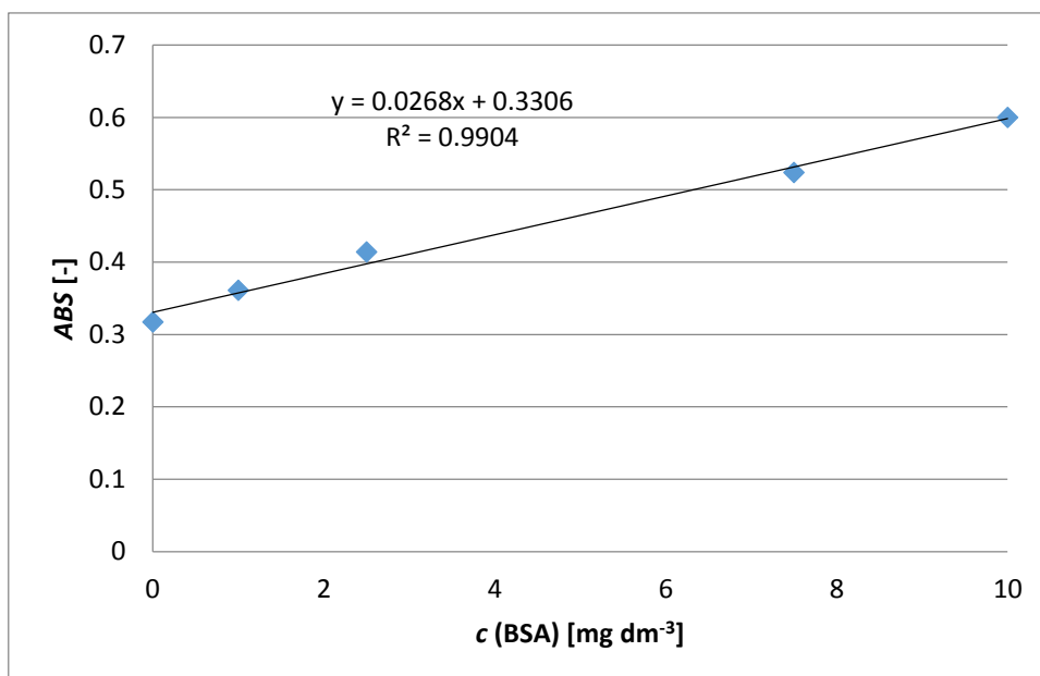
Slika 34. Baždarni diagram za određivanje koncentracije proteina ( c(\text{BSA}) = 0-10 \text{ mg dm}^{-3} ), \lambda = 595\text{nm} )
