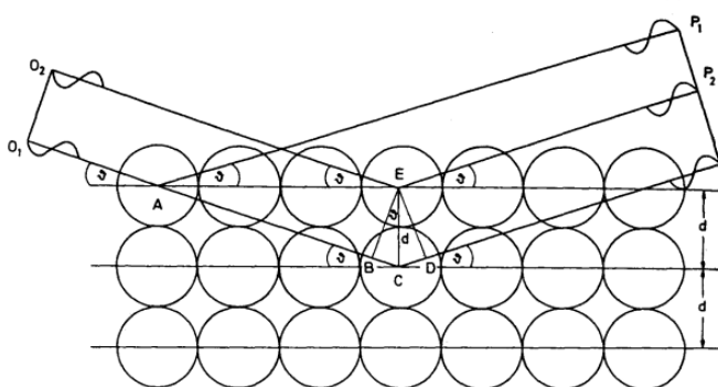
Slika 4. Shematski prikaz interferencije rendgenskih zraka [42]
