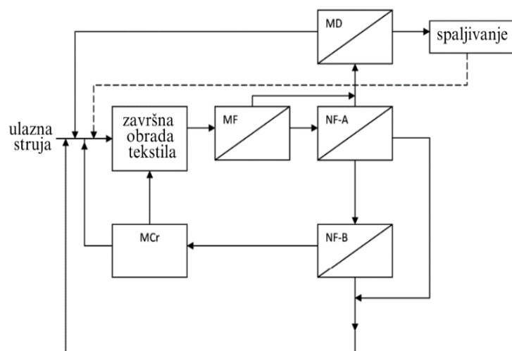
Slika 7. Integrirani model obrade otpadne vode (puna linija-vodeni tok, isprekidana linija-energetski tok); MF-mikrofiltracija, NF-nanofiltracija, MD- membranska destilacija, MC- membranska kristalizacija [17]
