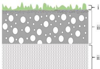
Slika 3. Poprečni presjek TFC membrane: i) poliamidni gornji sloj, ii) mikroporozni srednji, iiii) poliesterna mreža [10]
