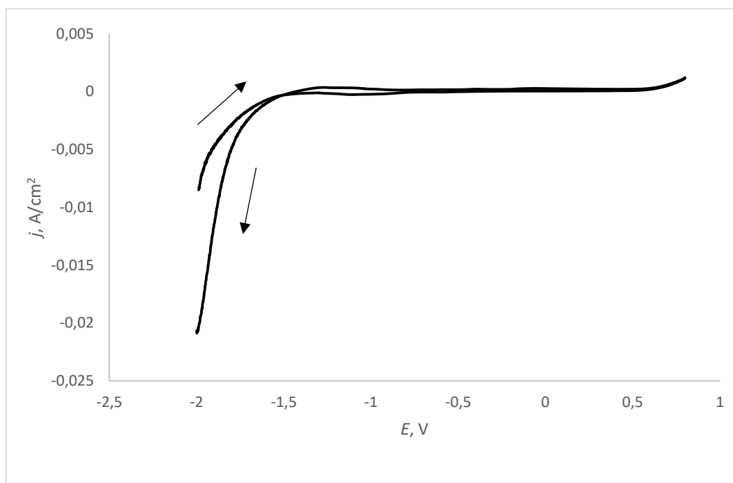
Slika 4.1. Ciklički voltamogram Zr elektrode u 1 mol dm -3 otopini NaOH uz brzinu promjene potencijala od 10 mV s -1
