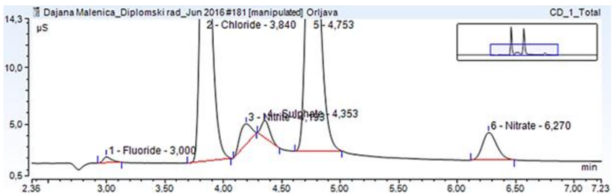
Slika 16. Kromatogram uzorka Orlijava dobiven IC analizom
