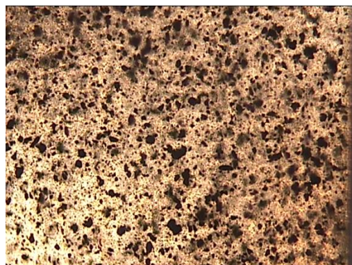
h) PU/MWCNT-COOH 2,0 %
