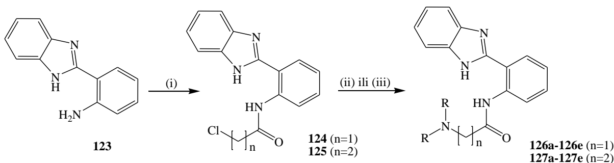
Shema 11. i) \text{Cl}(\text{CH}_2)_n\text{COCl} , \text{AcOH} , \text{AcONa} , r.t.; ii) \text{HNR}_2 , \text{DMF} , r.t., 24 h ( n = 1 ); iii) \text{HNR}_2 , \text{EtOH} , refl., 2 h ( n = 2 ).
