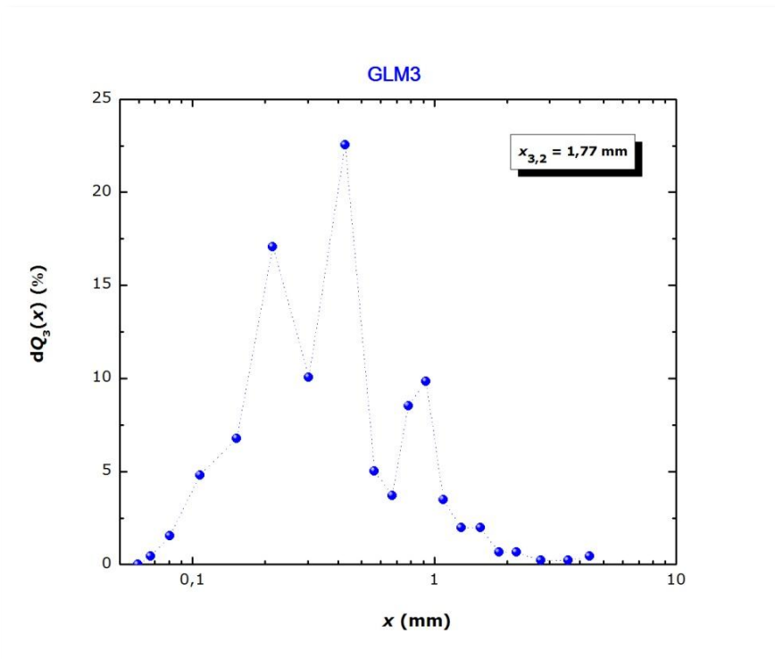
Slika 4.3. Grafički prikaz raspodjele veličina čestica laktoze monohidrata u granulatu GLM3.
