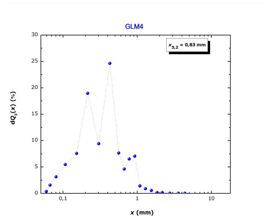
Slika 4.4. Grafički prikaz raspodjele veličina čestica laktoze monohidrata u granulatu GLM4.
