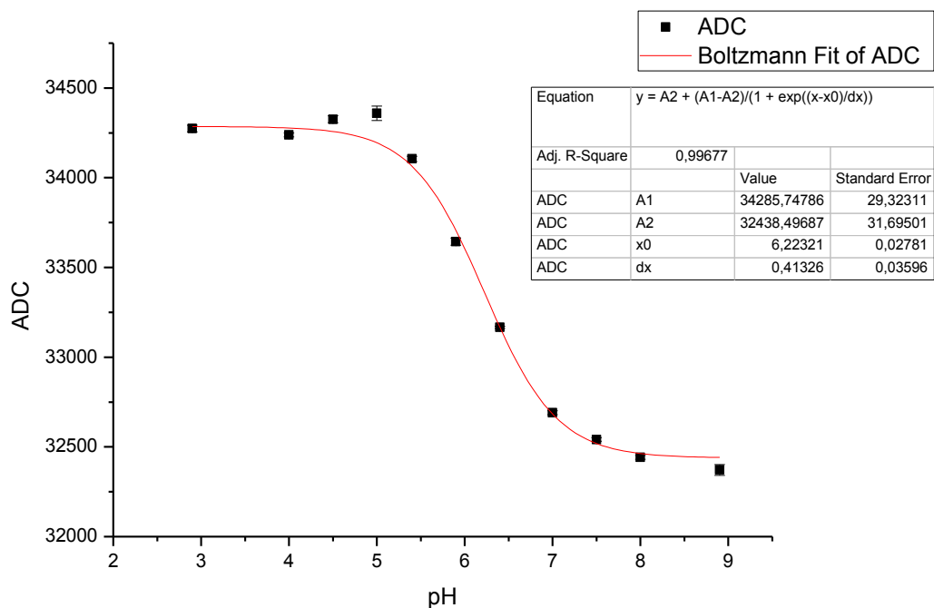
Slika 4.7. Grafički prikaz ovisnosti reflektiranog zračenja o pH dobiven uzastopnim mjerenjem micanjem kućišta
