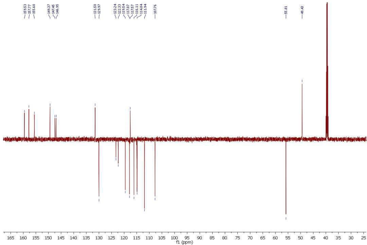
Slika 35. ^{13}\text{C} NMR spektar spoja 8e
