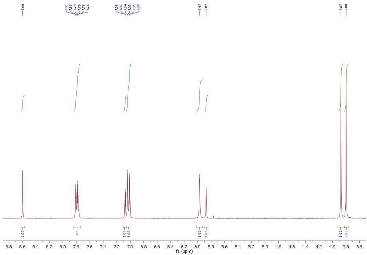
Slika 19. ^1\text{H} NMR spektar spoja 7b
