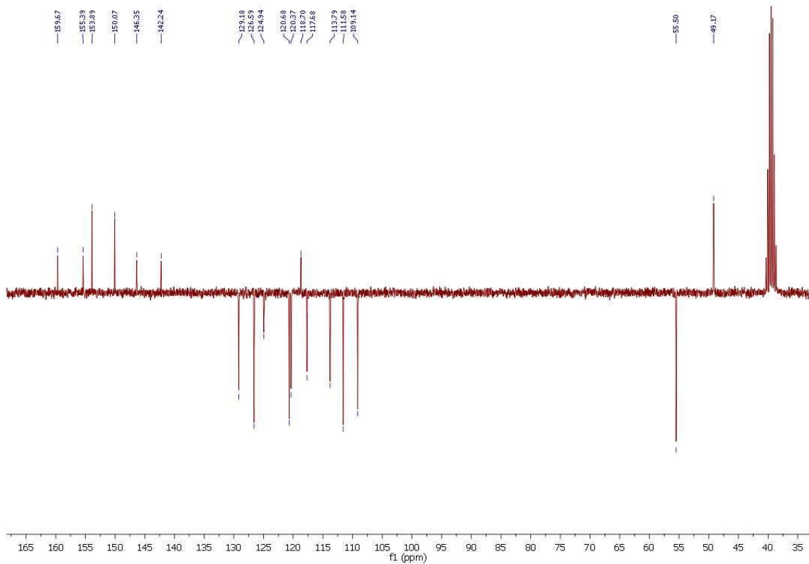
Slika 43. ^{13}\text{C} NMR spektar spoja 9d
