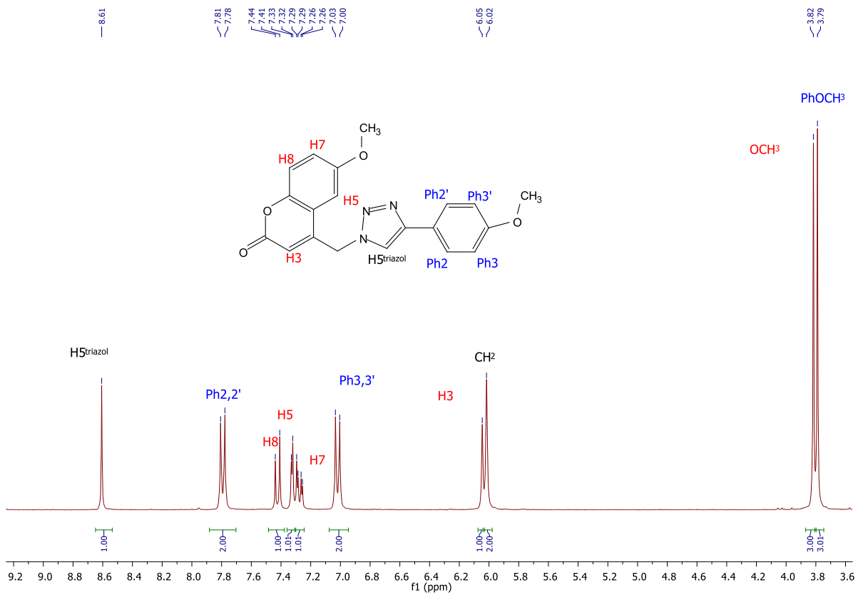
Slika 13. 1 H NMR spektar spoja 7b
