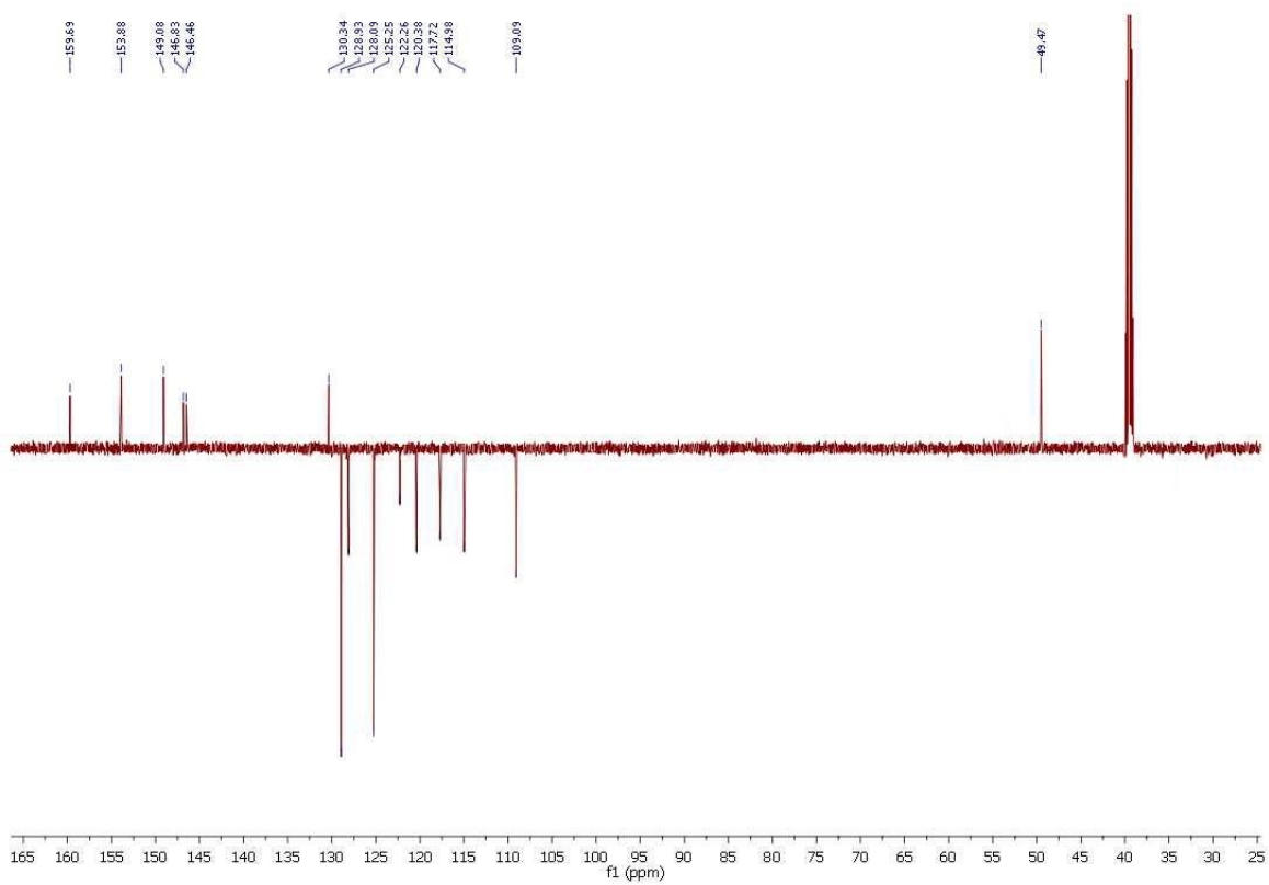
Slika 37. ^{13}\text{C} NMR spektar spoja 9a
