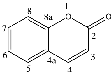
Slika 3. Struktura kumarina
