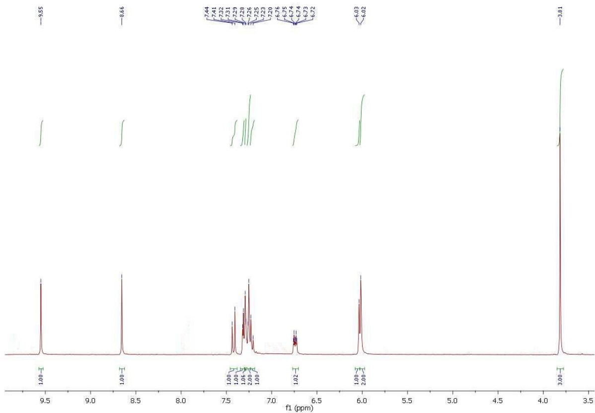
Slika 34. ^1\text{H} NMR spektar spoja 8e
