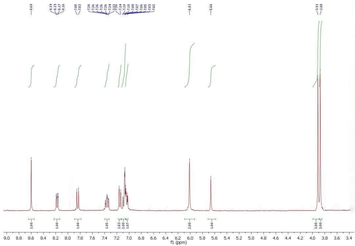
Slika 23. ^1\text{H} NMR spektar spoja 7d
