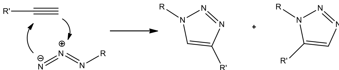
Slika 11. Huisgenova 1,3-dipolarna cikloadicija
