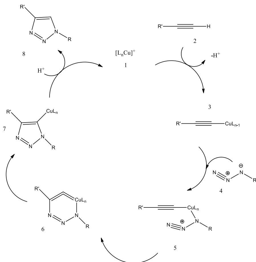
Slika 11. Mehanizam 1,3-dipolarne cikloadicije kazalirane Cu (I) ionima
