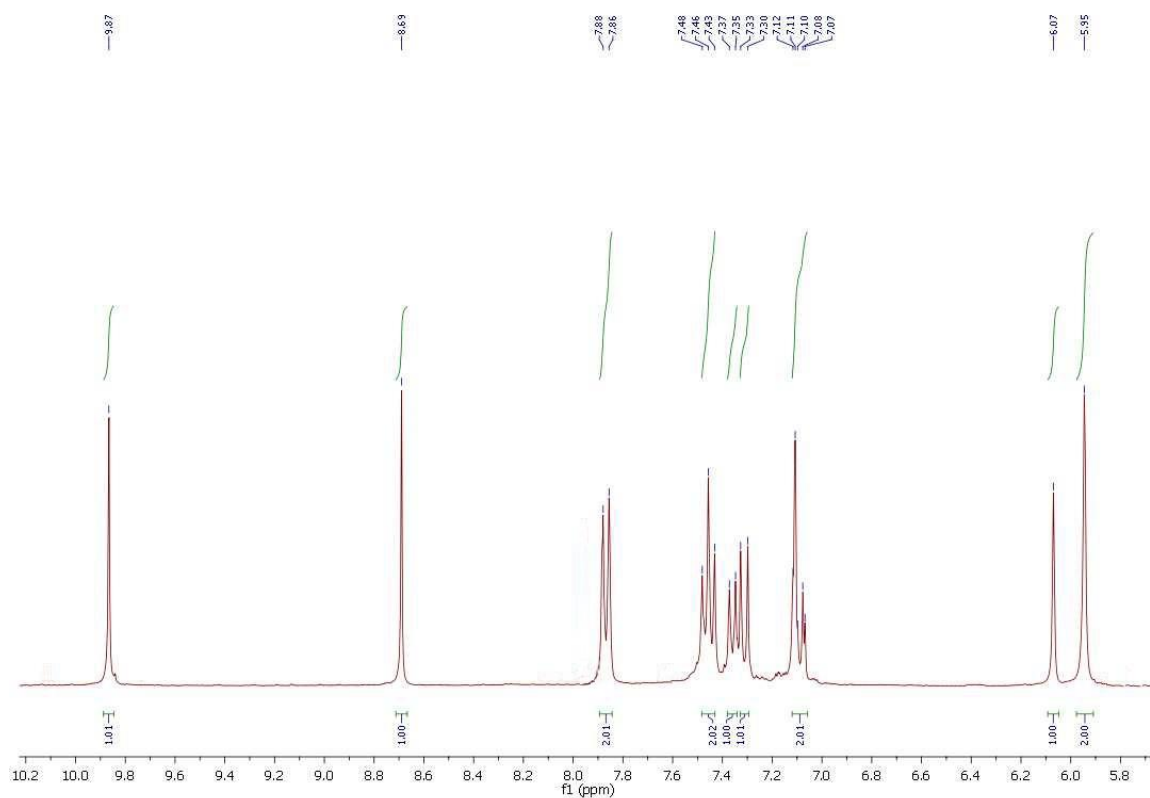
Slika 36. ^1\text{H} NMR spektar spoja 9a
