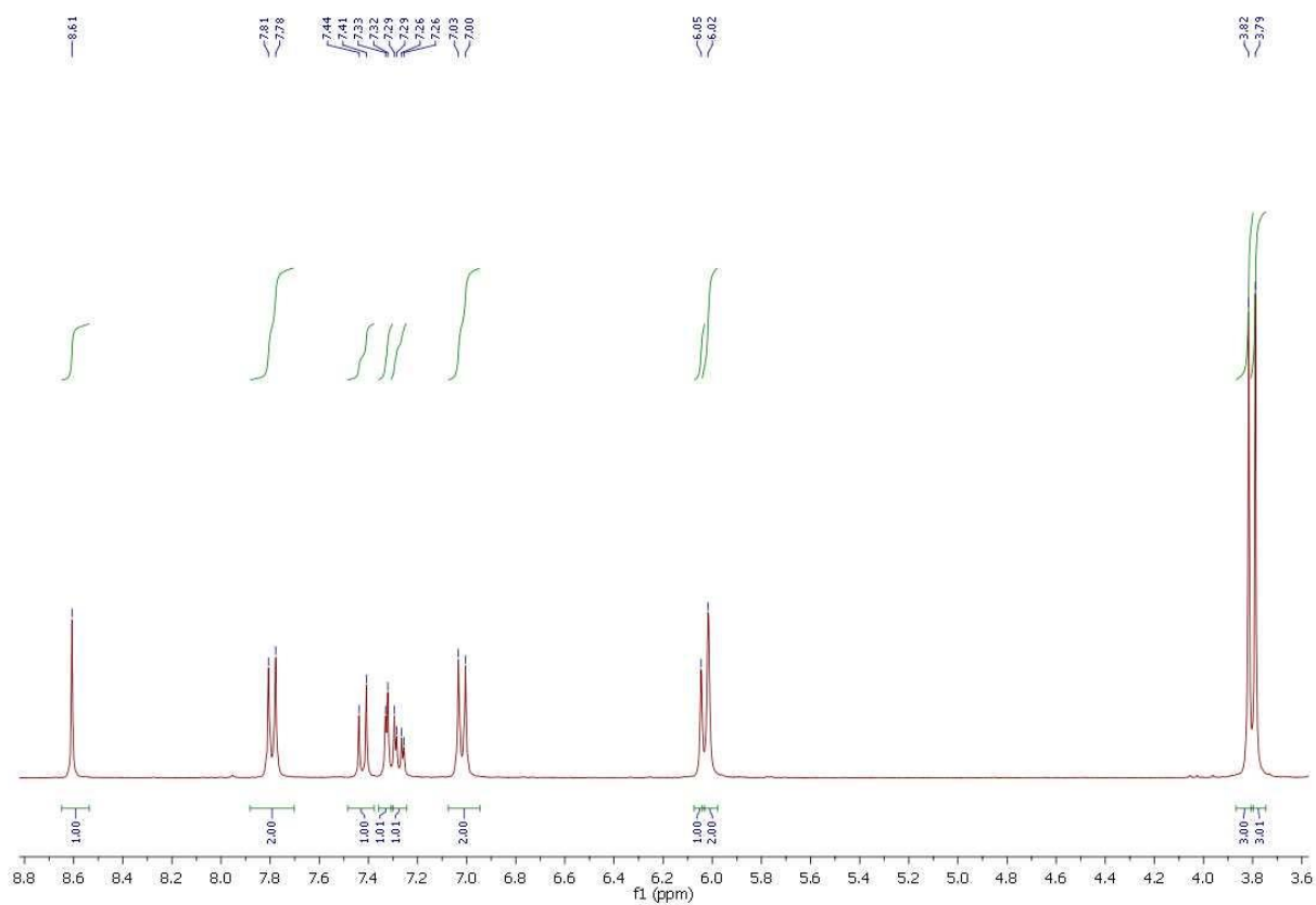
Slika 28. ^1\text{H} NMR spektar spoja 8b
