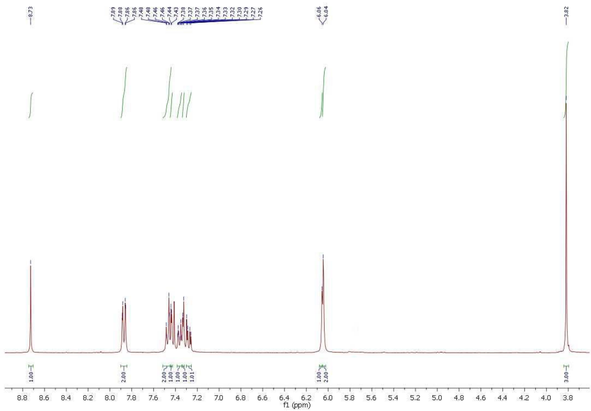
Slika 26. ^1\text{H} NMR spektar spoja 8a
