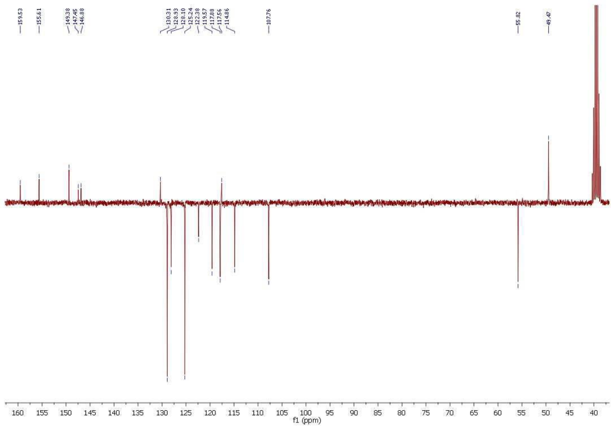
Slika 27. ^{13}\text{C} NMR spektar spoja 8a
