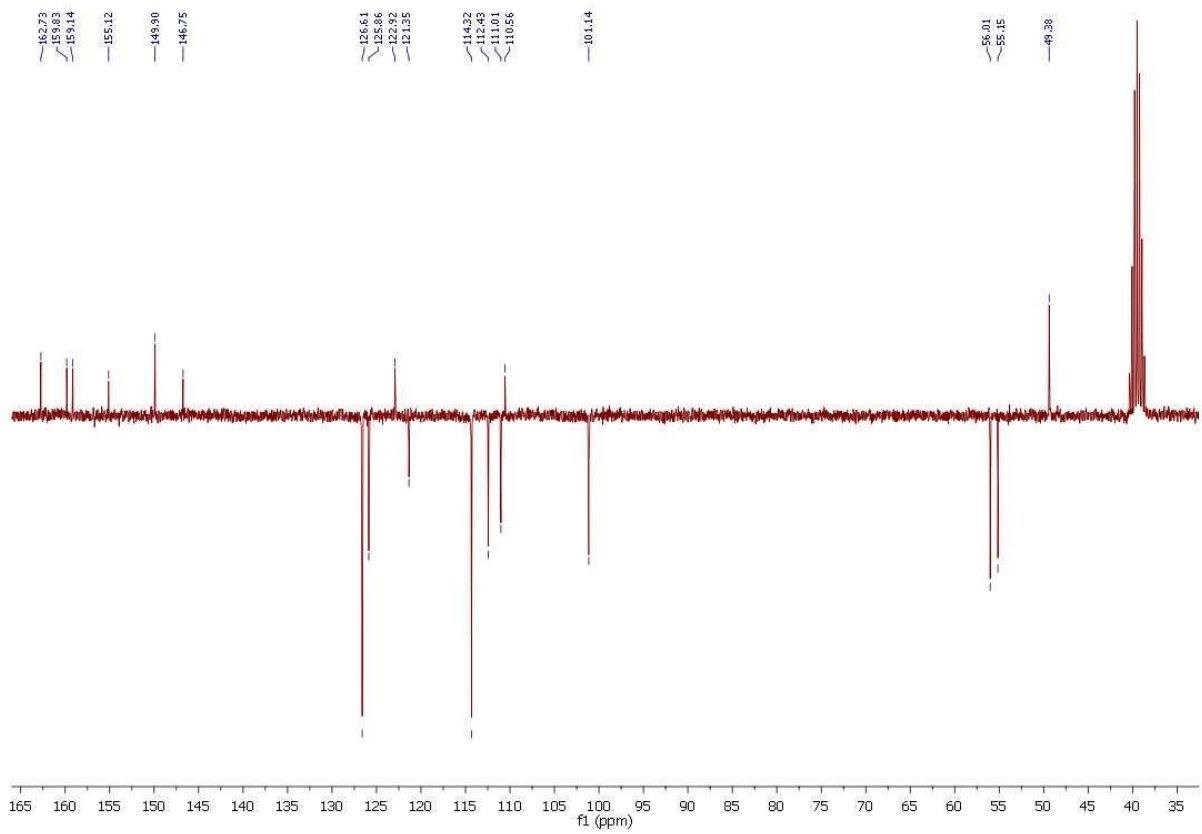
Slika 20. ^{13}\text{C} NMR spektar spoja 7b
