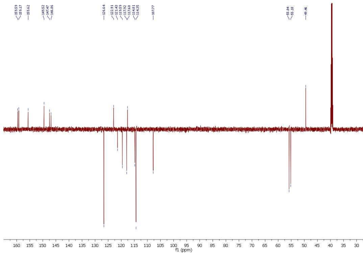
Slika 29. ^{13}\text{C} NMR spektar spoja 8b
