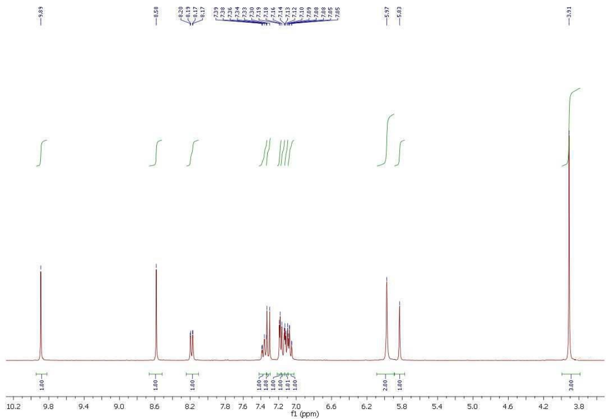
Slika 42. ^1\text{H} NMR spektar spoja 9d
