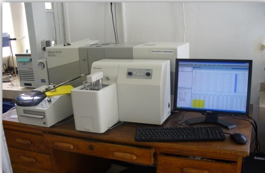
Slika 3.4. Fotografija uređaja za određivanje raspodjele veličina čestica metodom laserske difrakcije SALD-3101 (Shimadzu, Kyoto, Japan) (Fakultet kemijskog inženjerstva i tehnologije, Zavod za mehaničko i toplinsko procesno inženjerstvo, Zagreb, Republika Hrvatska).
