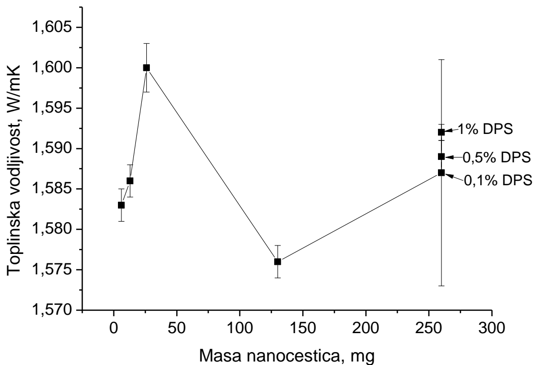
Slika 4.6.2. Promjena toplinske vodljivosti P4DPS nanofluida, 2. dan
