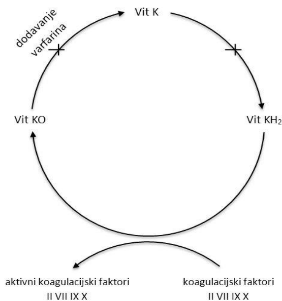
Schema 12. Ciklus varfarina i vitamina K
