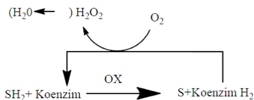
SLIKA 2. Djelovanje oksidaze
