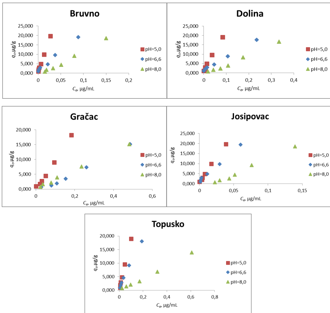
Slika 22. Linearne sorpcijske izoterme febantela za ispitivane uzorke tla pri različitim pH uvjetima: pH=5,0, pH=6,6 i pH=8,0
