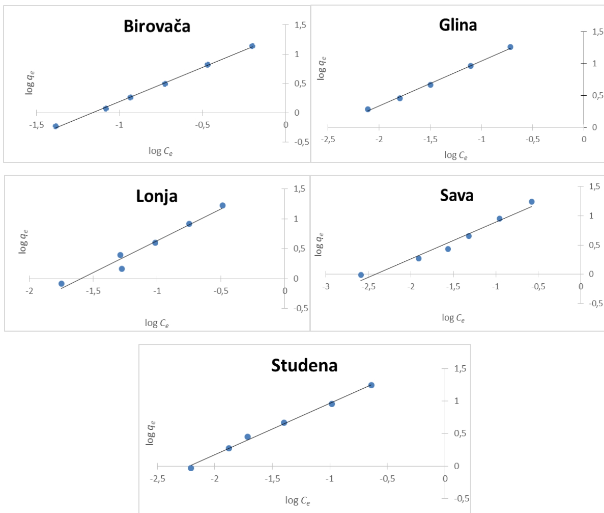
Slika 17. Grafički prikaz Freundlichovih sorpcijskih izoterma febantela za ispitivane sedimente pri 0,01 M \text{CaCl}_2
