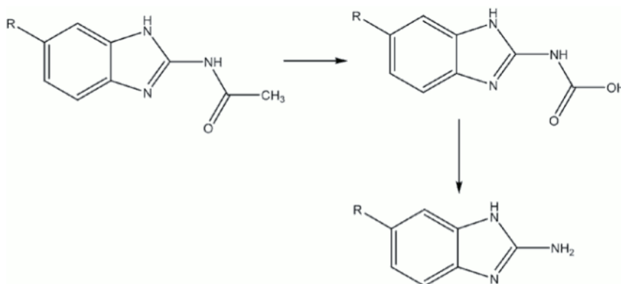
Slika 2. Fotorazgradnja benzimidazolnih anthelmintika [10]
