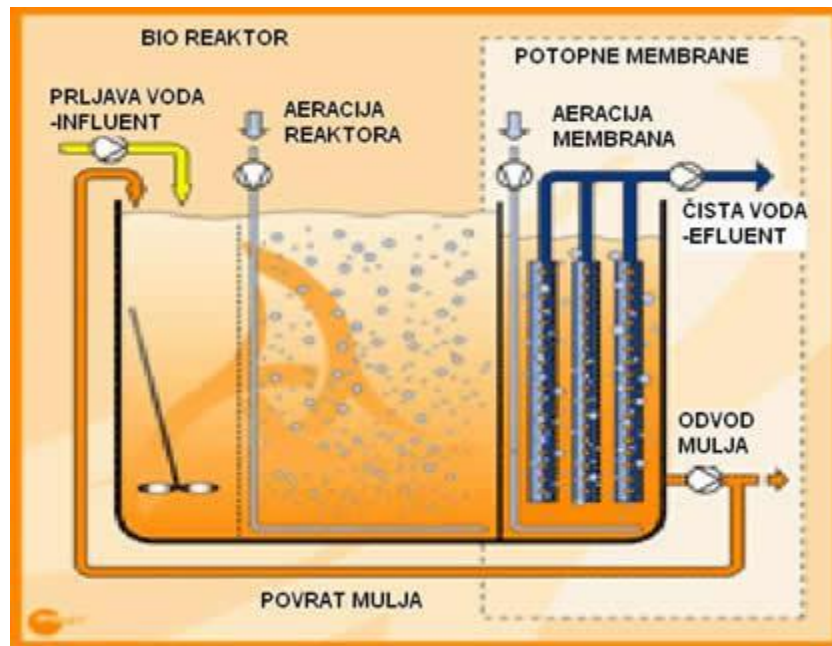
Slika 8. Shematski prikaz membranskog bioreaktora [1]
