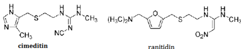
Slika 5. Kemijska struktura cimetidina i ranitidina [1]
