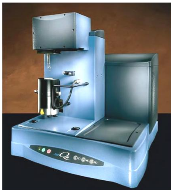
Slika 28. Termogravimetar TA Instruments Q500
