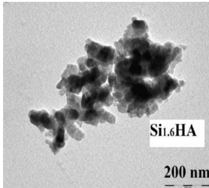
Slika 7. TEM mikrograf SiHA sinteriranog na 900°C.
