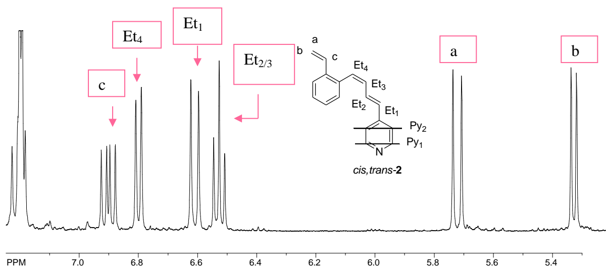
Slika 11. Aromatski dio 1 H NMR spektra cis,trans - 2 .
