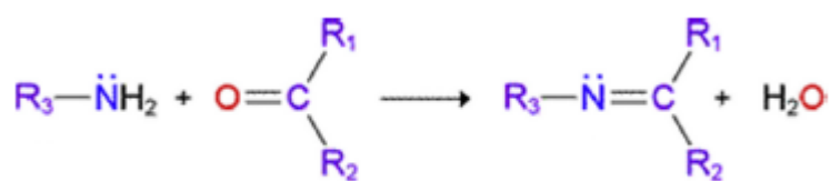
Slika 6. Shematski prikaz sinteze Schiffove baze reakcijom primarnog amina sa aldehidom ili ketonom [21]
