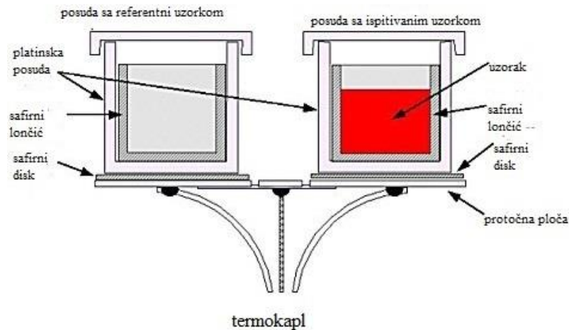
Slika 11. DSC s toplinskim tokom 12 .
