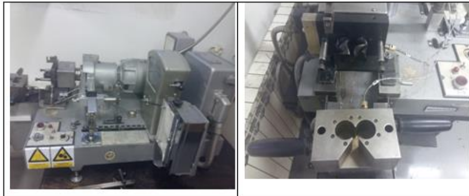
Slika 13. Brabender gnjetilica.
