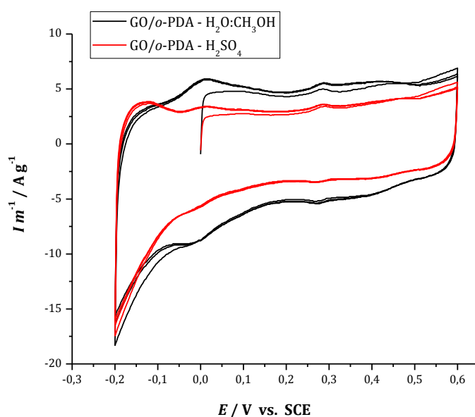
Slika 4.9. Rezultati ispitivanja (po 3 ciklusa) GO-elektroda inkubiranih u 0,1 M otopinama o -PDA (1 M otopina H_2SO_4 i H_2O:CH_3OH (9:1) otopina) u 1 M H_2SO_4 kao elektrolitu i pri brzini promjene potencijala od 50 mV/s.
