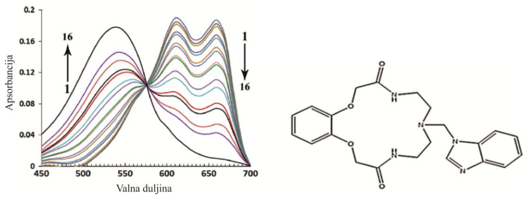
Slika 7. ApSORPCIJSKI spektri optode za detekciju iona srebra od najmanje koncentracije - 1 do najviše - 16.i struktura korištenog derivata benzimidazola u ulozi ionofora. 8
