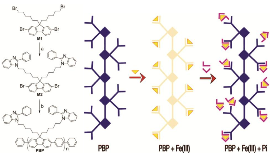
Slika 8. Koraci pri sintezi polifulerena te senzorski mehanizam gdje se fluorescencija gasi pri vezanju Fe 3+ , a pri vezanju fosfata, uslijed izmiještanja Fe 3+ , fluorescencija se obnavlja s povećanjem intenziteta od 106%. 32
