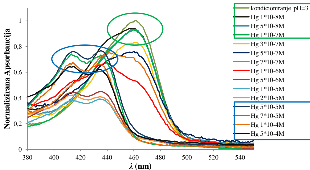
Slika 30. Apsoorbcijski spektri odziva optode na \text{Hg}^{2+} s rasponom koncentracija od c = 5 \cdot 10^{-4} M do c = 1 \cdot 10^{-8} M.
