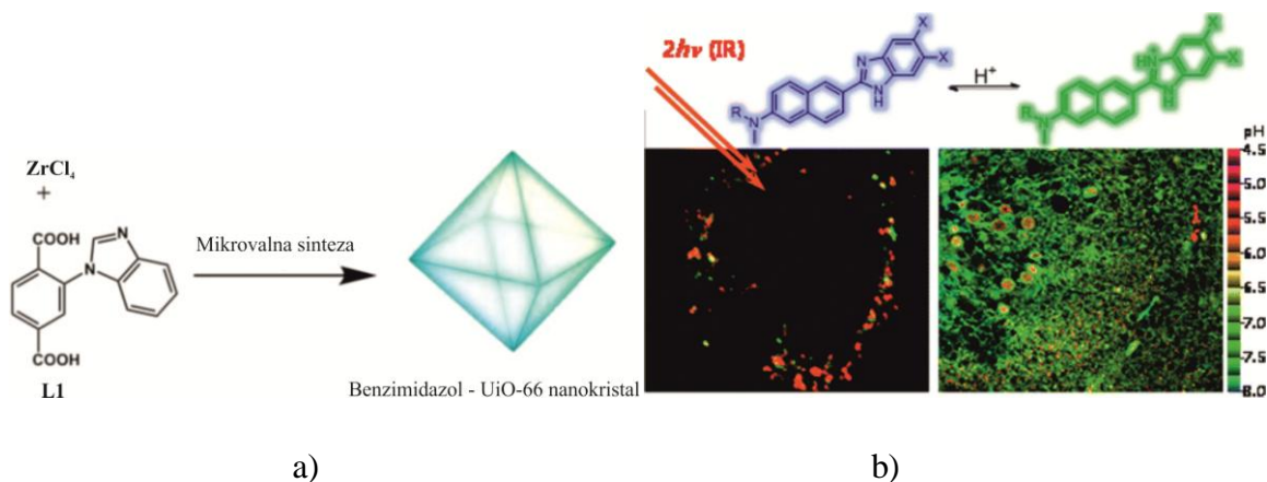
Slika 5. a) Sinteza benzimidazolnog funkcionalnog materijala UiO-66, b) Ratiometrijska dvofotonska proba pripremljena iz derivata benzimidazola za praćenje kiseline u živim stanicama i tkivima s prijelazom emisije u području plavo - zeleno u ovisnosti o kiselosti, u rasponu pH od 4,9 do 6,1. 29, 30
