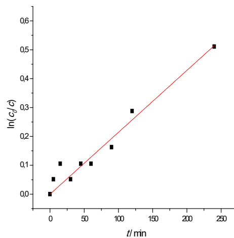
Slika 35. Kinetyka razgradnje na uzorku FM3
