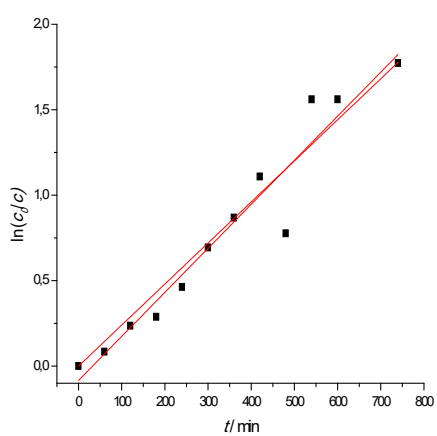
Slika 34. Kinetyka razgradnje na uzorku FK6, 12 h
