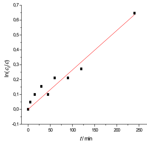
Slika 33. Kinetyka razgradnje na uzorku FK6, 4h
