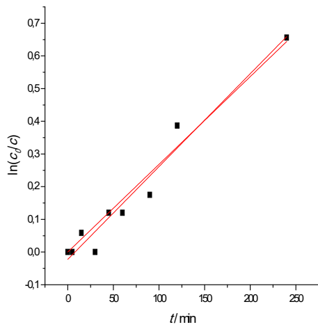
Slika 32. Kinetyka razgradnje na uzorku FK5t
