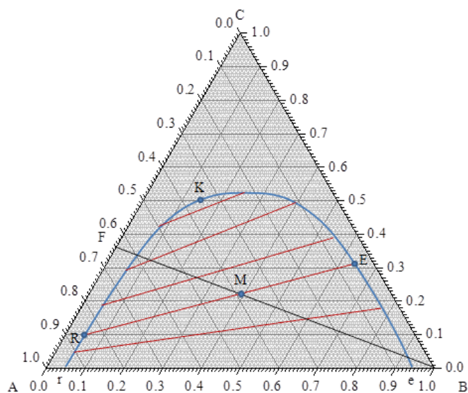
Slika 2.2. Ravnoteža kapljevina–kapljevina
