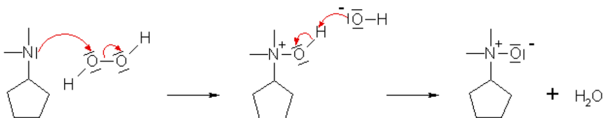
Slika 6. Mehanizam reakcije tercijarnog amina s \text{H}_2\text{O}_2
