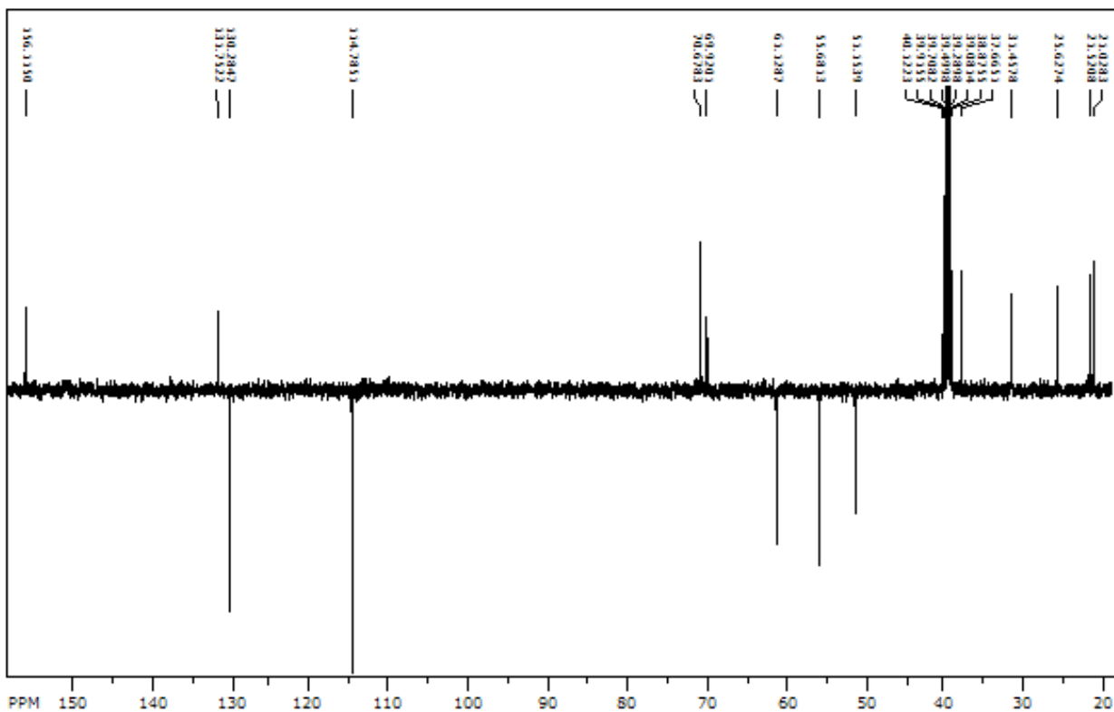
Prilog 3. ^{13}\text{C} NMR spektar aromatskog N-oksida terciarnog amina A
