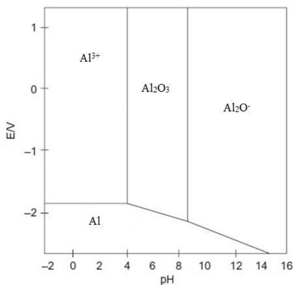
Slika 9. Pourbaixov dijagram aluminijske površine u vodenim otopinama pri 25°C [16].
