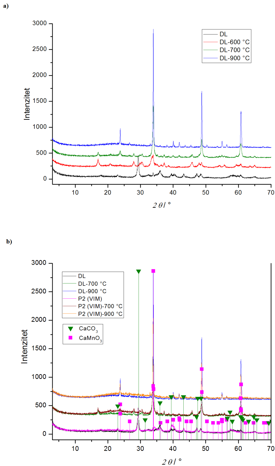
Slika 14. Rezultati rendgenske analize: a) Usporedba uzoraka dobivenih limunskom metodom pri različitim temperaturama žarenja, b) Usporedba uzoraka dobivenih limunskom metodom sa različitim omjerom limunske kiseline (P2 (VIM)) 18 pri različitim temperaturama žarenja
