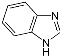
Slika 6. Struktura molekule benzimidazola
