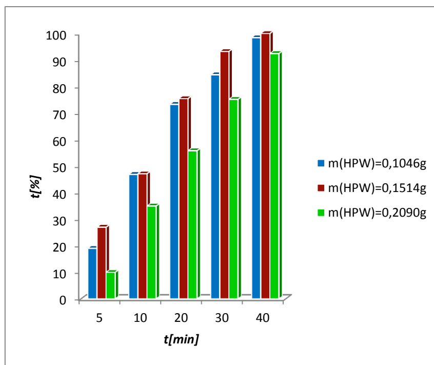
Slika 25. Konverzije DBT-a u ovisnosti o masi katalizatora i vremenu reakcije ( T = 50^{\circ}\text{C} , uzv=70 W, 80 %)
