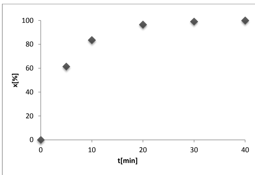
Slika 33. Konverzija DBT-a u ovisnosti o vremenu reakcije u procesu oksidacije ( T=70^{\circ}\text{C} , \text{O:K}=22,18:1 )
