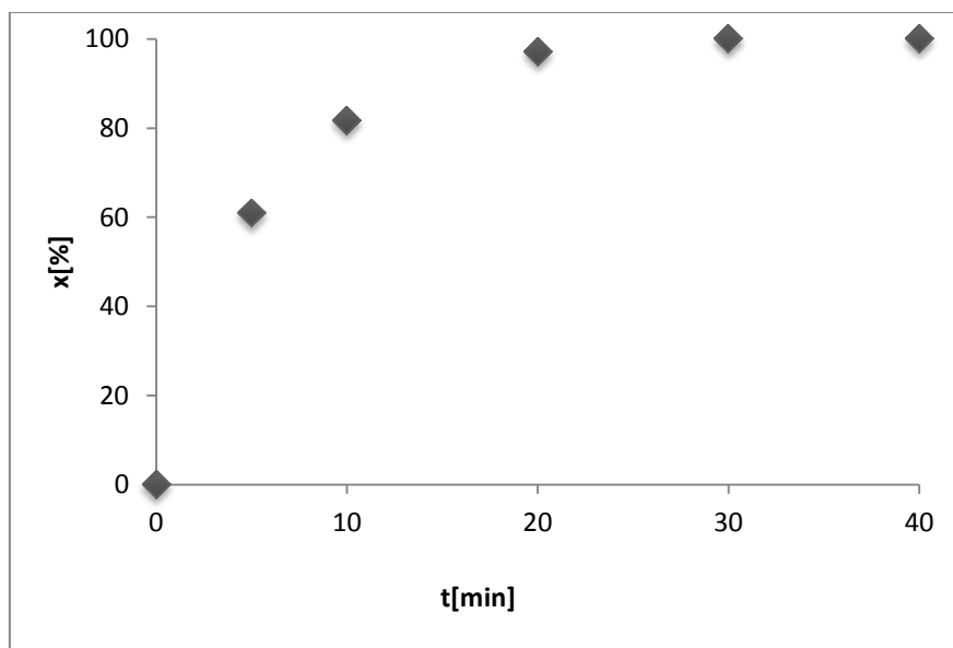
Slika 32. Konverzija DBT-a u ovisnosti o vremenu reakcije u procesu oksidacije ( T=70^{\circ}\text{C} , \text{O:K}=22,18:1 )
