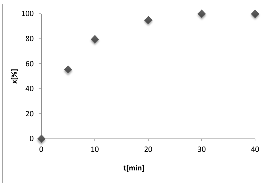
Slika 31. Konverzija DBT-a u ovisnosti o vremenu reakcije u procesu oksidacije ( T=70^{\circ}\text{C} , \text{O:K}=22,18:1 )
