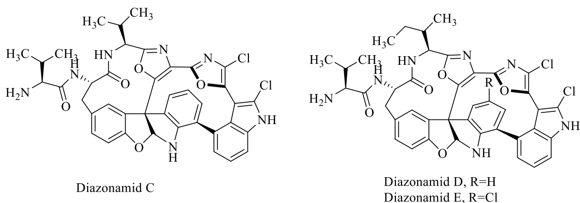
Slika 13. Struktura diazonamida.
