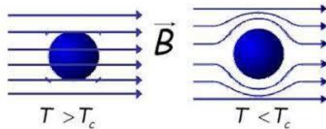
Slika 1.2. Magnetske silnice kada je temperatura T viša od kritične temperature T_c , i magnetske silnice kada je temperatura T niža od kritične temperature T_c .
